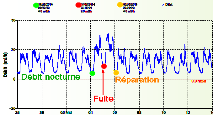
Suivi par le SEAPaN des débits d'eau potable à l'aval de Coarrazze
